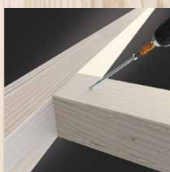
Hoofdhulpligger verbinding
